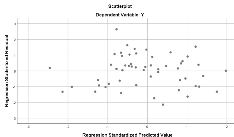
Gambar 2. Heteroskedastisitas (Scatterplot)
